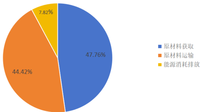
10KV管母线碳排放量kgCO 2 e/米
